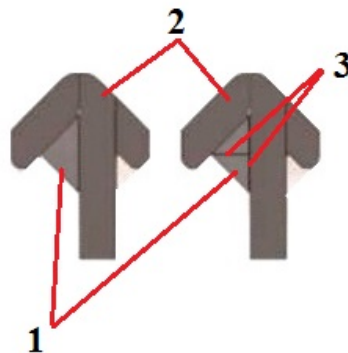
Рис. 2 Рекомендований спосіб визначення центру заготовки 1 – заготовка; 2 – пристосування; 3 – лінії для визначення центру
